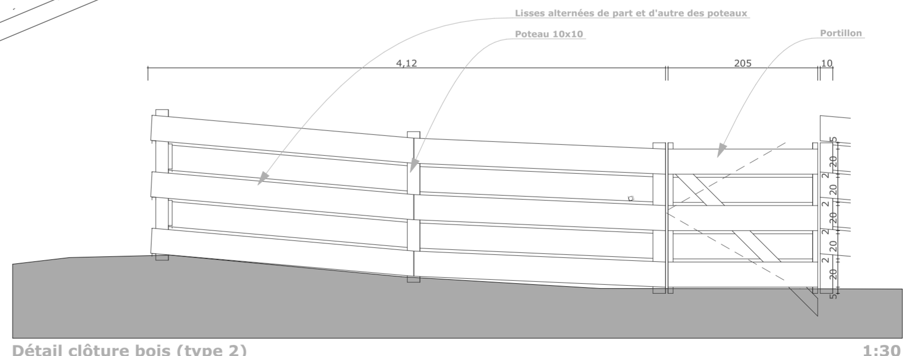
Détail clôture bois (type 2)
